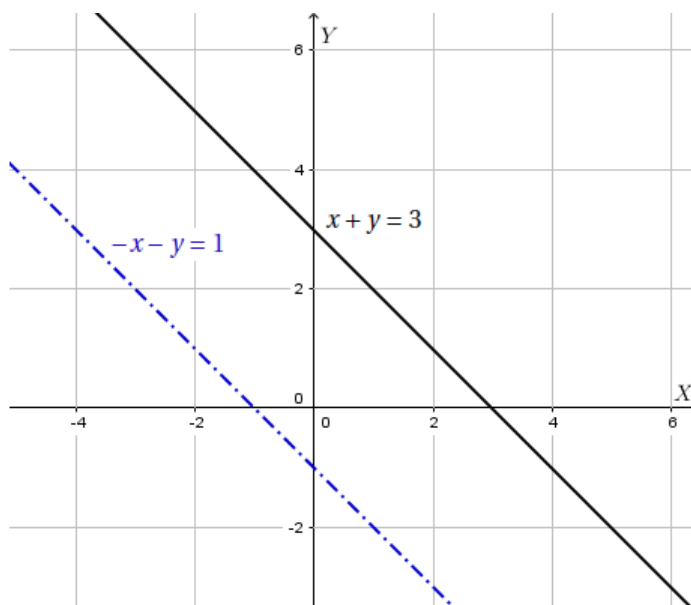
Figura 5: Interpretação geométrica da solução de um sistema impossível, onde se observa que, para essa situação, as retas são paralelas.
